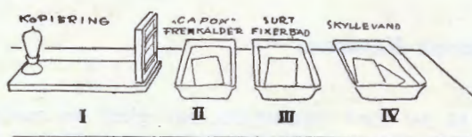
Fig. 2. „Capox“ Processens fire Trin.
