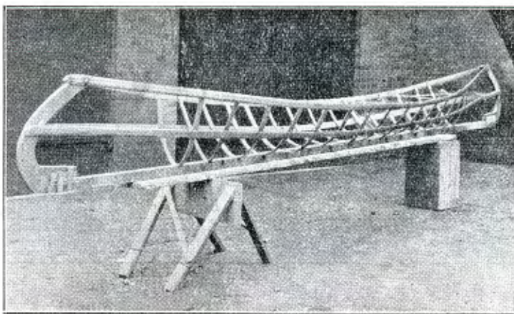
Skelet til en 4 m Kano
