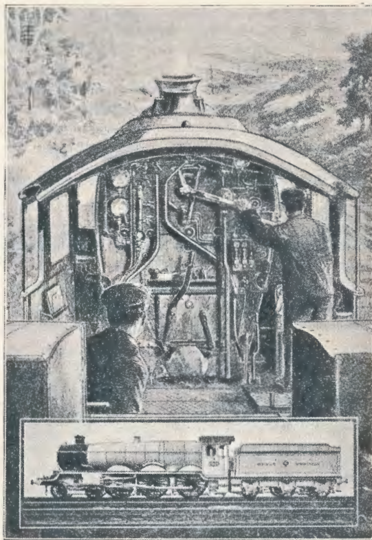
Paa Fyrpladsen paa »Den flyvende Skotte« i fuld Fart. Forneiden ser man et Billede af Lokomotivet selv
