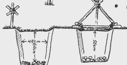
DETTE ER DET ABSOLUT MINDSTE MÅL PÅ AFFALDSHUL OG FÆTTFÆLDE, HVIS I VIL BEVARE HYGIEJEN I LEJREN
