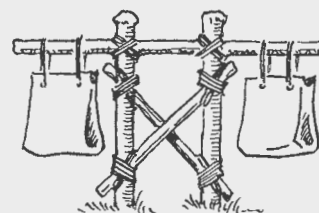
VANDSÆKKENE MÅ IKKE STÅ PÅ JORDEN
