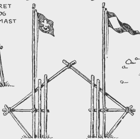
EN FLOT INDGANGSPORTAL
