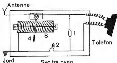
Set fra oven
