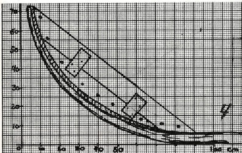
4. stævprofil (det skraverede borthøvles efter oplimningen).
