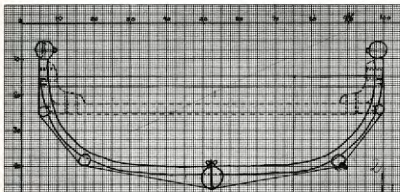
2. tværsnit og spanterids.
